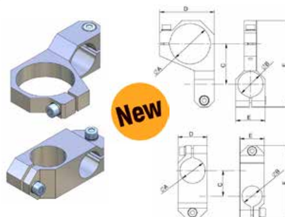
Cross Connector Tube Kreuzklemmstück Rohr Connessione a Croce Tubo Bloc de Conexion en Croix Pieza de Apriete en Cruz
