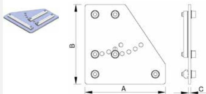
Corner Joint Plate Eckverbinder Connessione Angolare Bride à Angle Elemento de Unión en Ángulo
