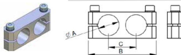
Parallel Clamp Parallelklemmstück Staffa parallela Soporte Paralelo
